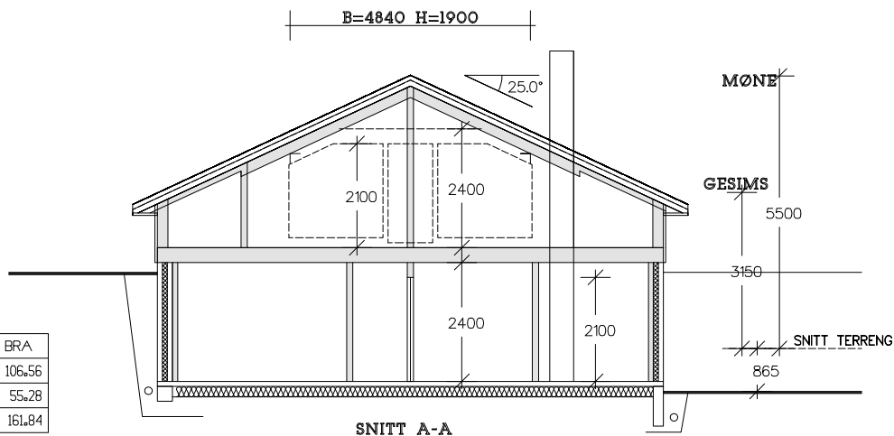
SNITT A-A
